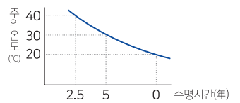
콘덴서수명(24시간/일 사용)
